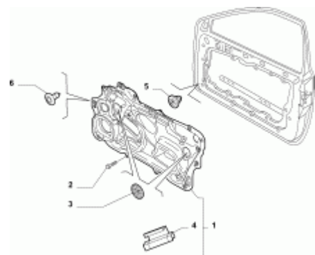
70129/10 - SIDE FRONT DOORS (Var.:2/Rev.:0)
